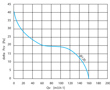
Charakterystyka wydajności wentylatora Fan efficiency characteristic
